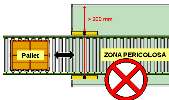
Protezione meccanica non corretta
