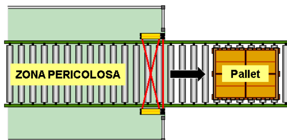
L raggi incrociati in uscita
