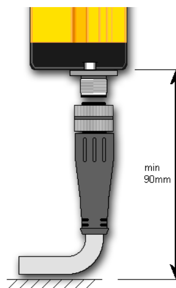
M12 diritto
