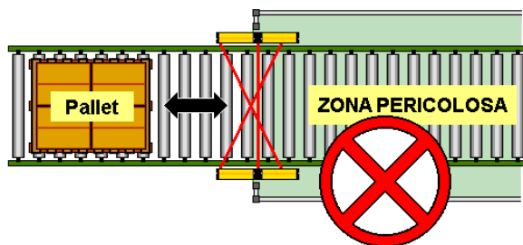
Errato orientamento T raggi incrociati
